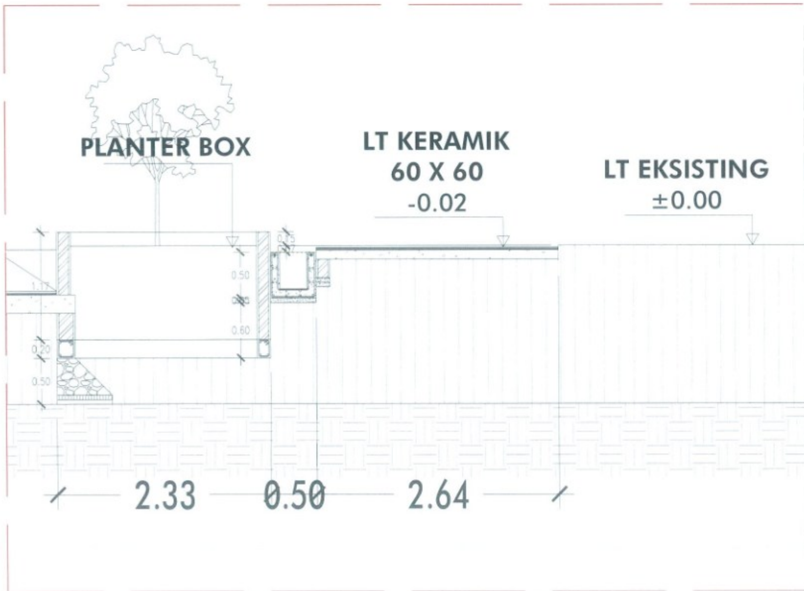
POTONGAN B-B SKALA 1:80
