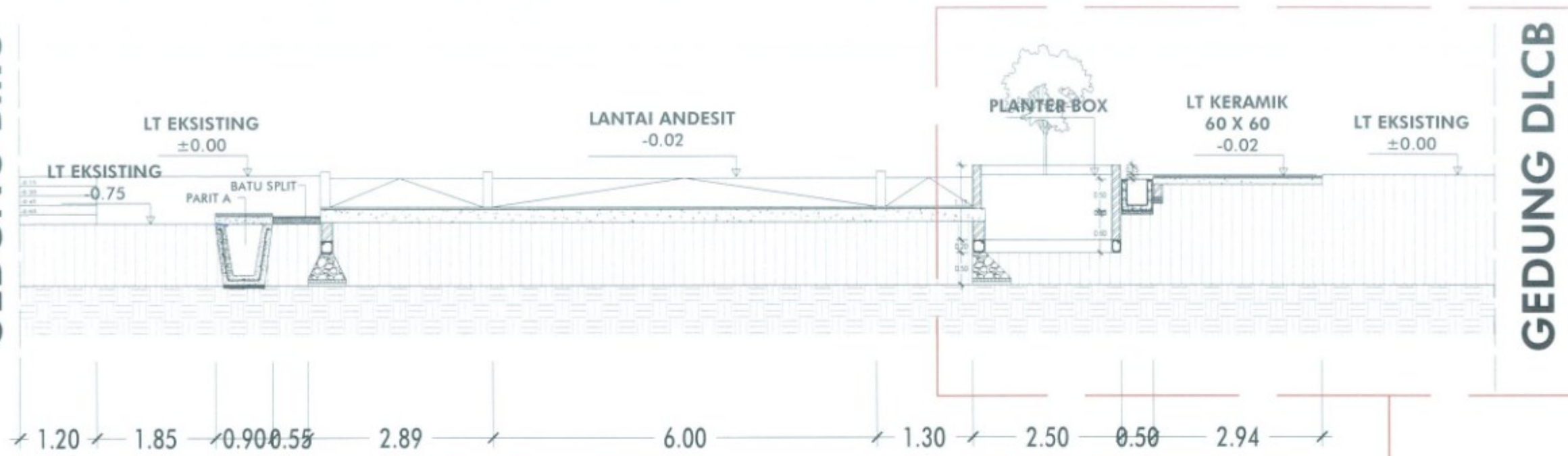
POTONGAN B-B SKALA 1:80
